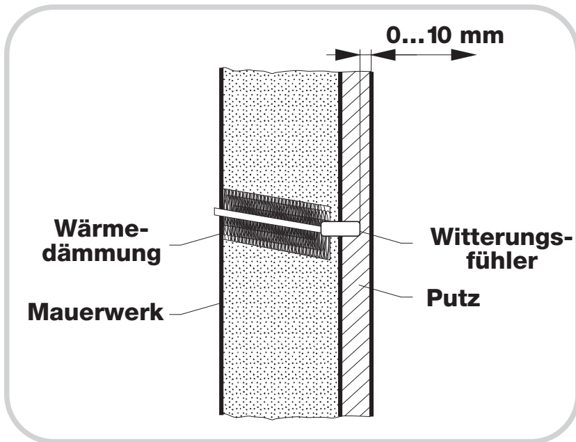
Übliche Lage des Witterungsfühlers in einer Außenwand.
